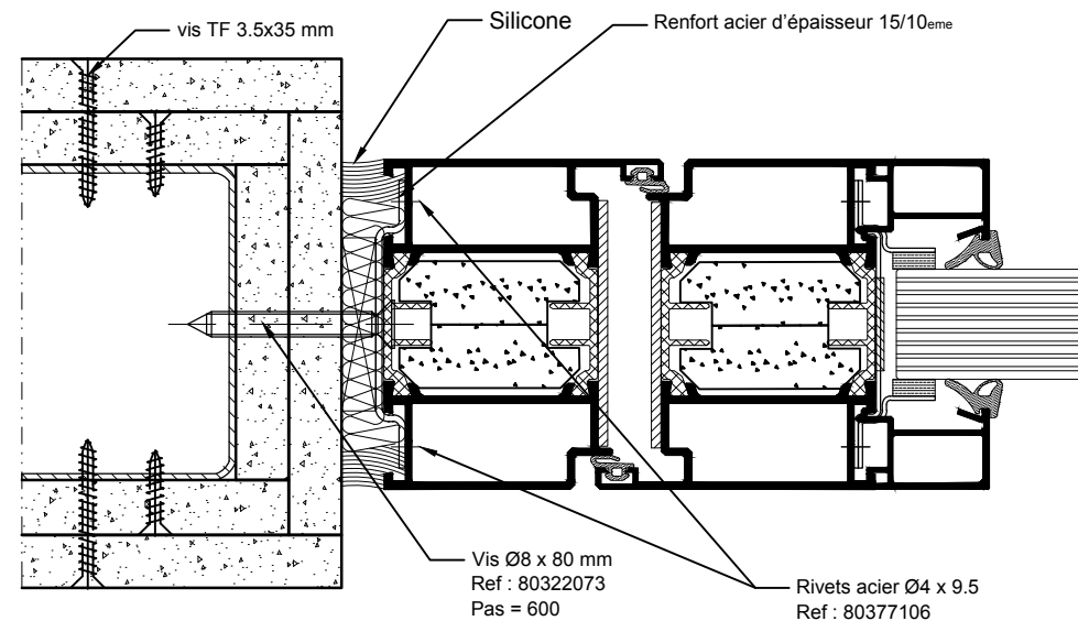
Montée en cloison légère T 126/2
