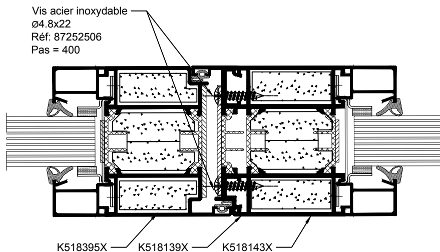
Montée en cloison EMV T 126/2
